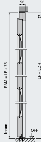
Nebentür aus Massivholz Einbau in der Öffnung
