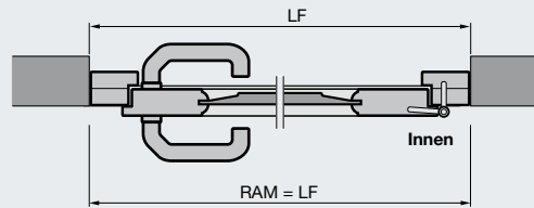
Nebentür aus Massivholz Einbau in der Öffnung
